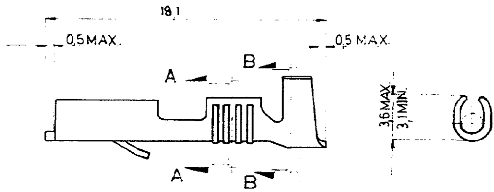
SECCION-A-A
