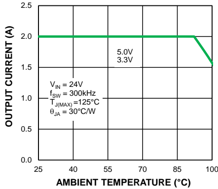
24V Input Thermal Derating MIC28512-1
