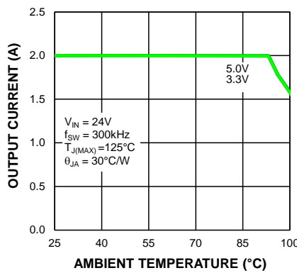
24V Input Thermal Derating MIC28512-2
